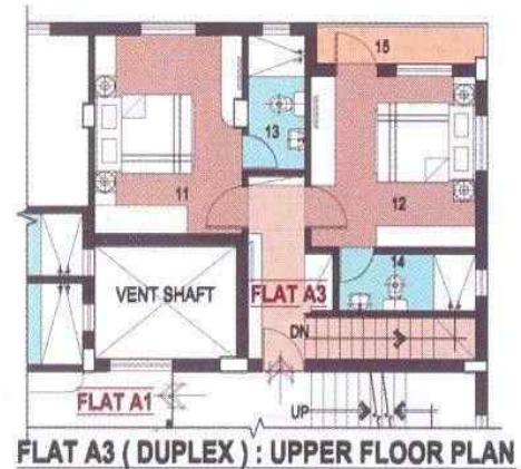
FLAT TYPE A3 [ DUPLEX ]
